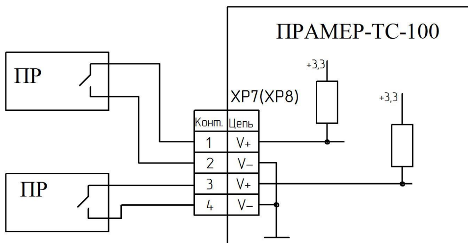
Рисунок 12 – Подключение ПР
